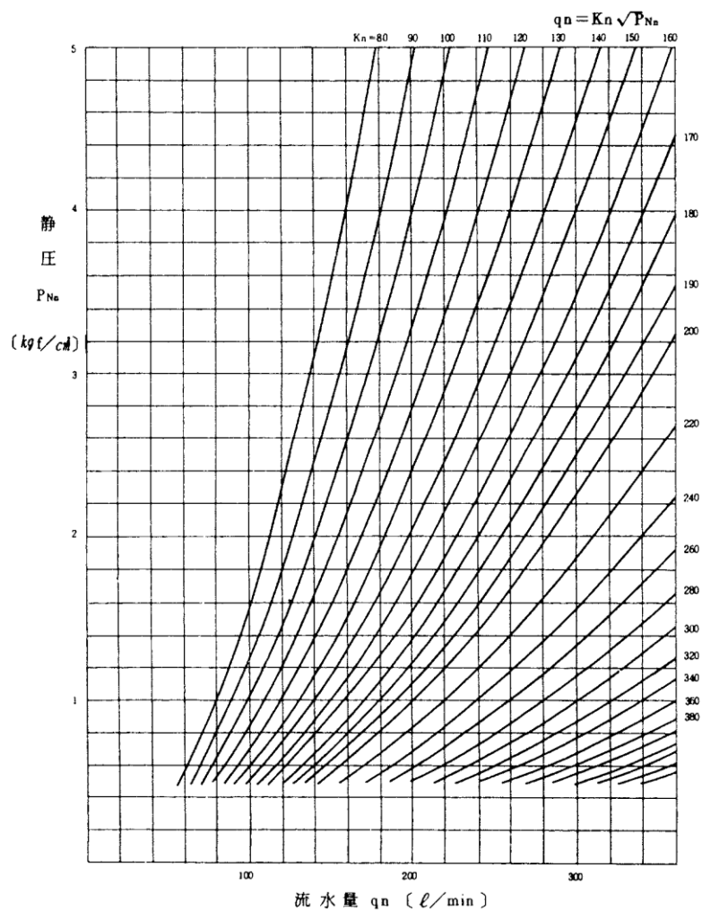
図3-10 流水表
