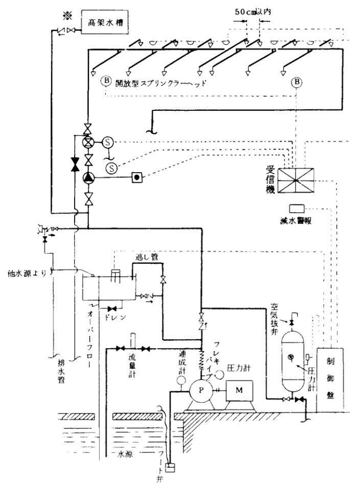
図3-4 開放型スプリンクラー設備の構造図例
