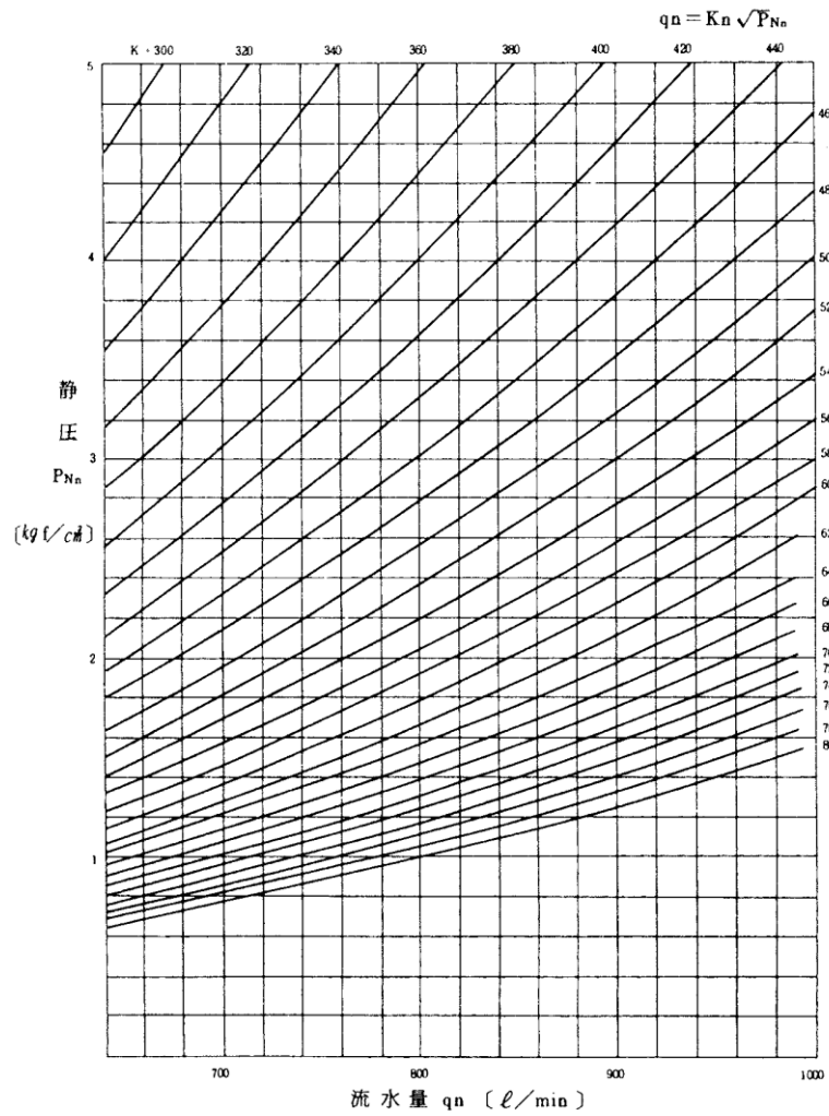
図3-12 流水表
