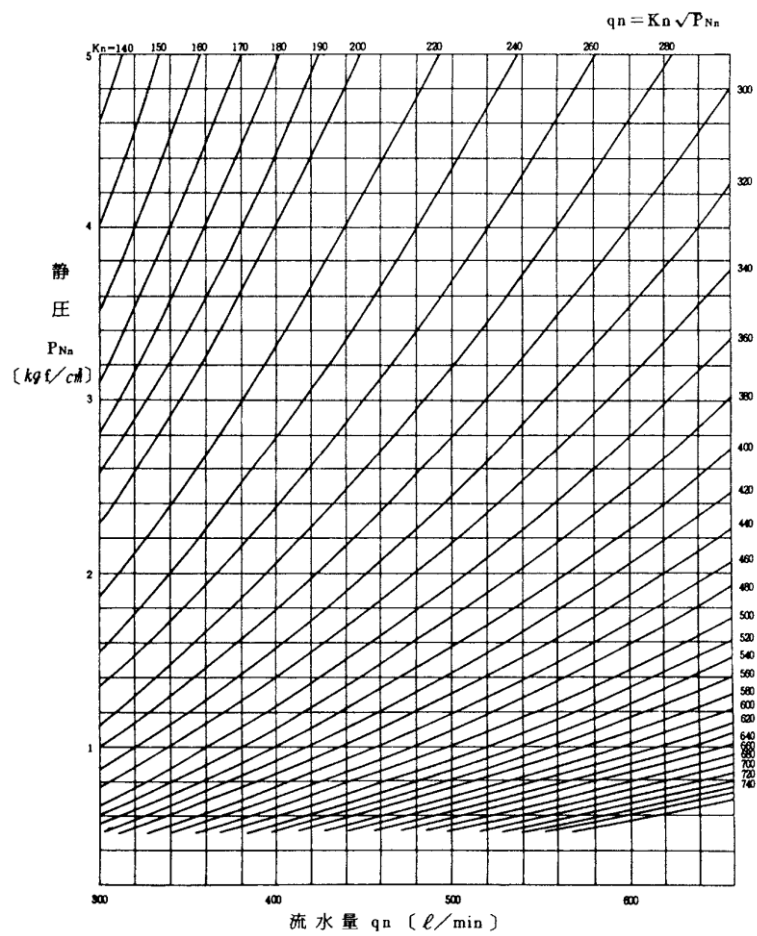
図3-11 流水表
